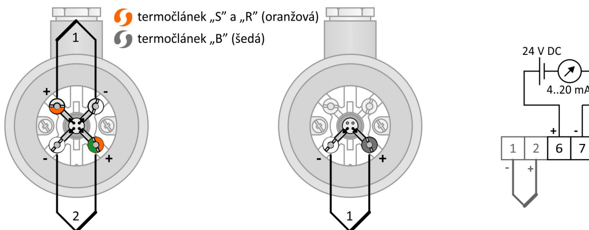
Obrázek 5MA.6: zapojení dvojitého termočláнку
